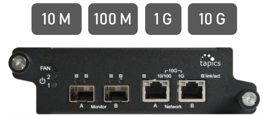
TAP 1 lien cuivre TACU1-10G
